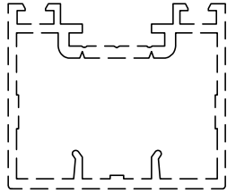
11-2512 Стойка одинарного остекления 100 мм
